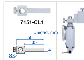
soporte de reloj comparador (opcional)
